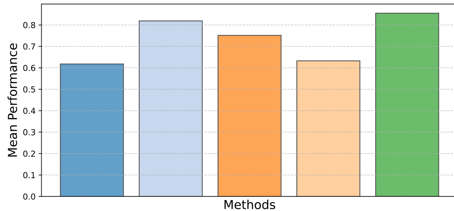
ROC AUC
