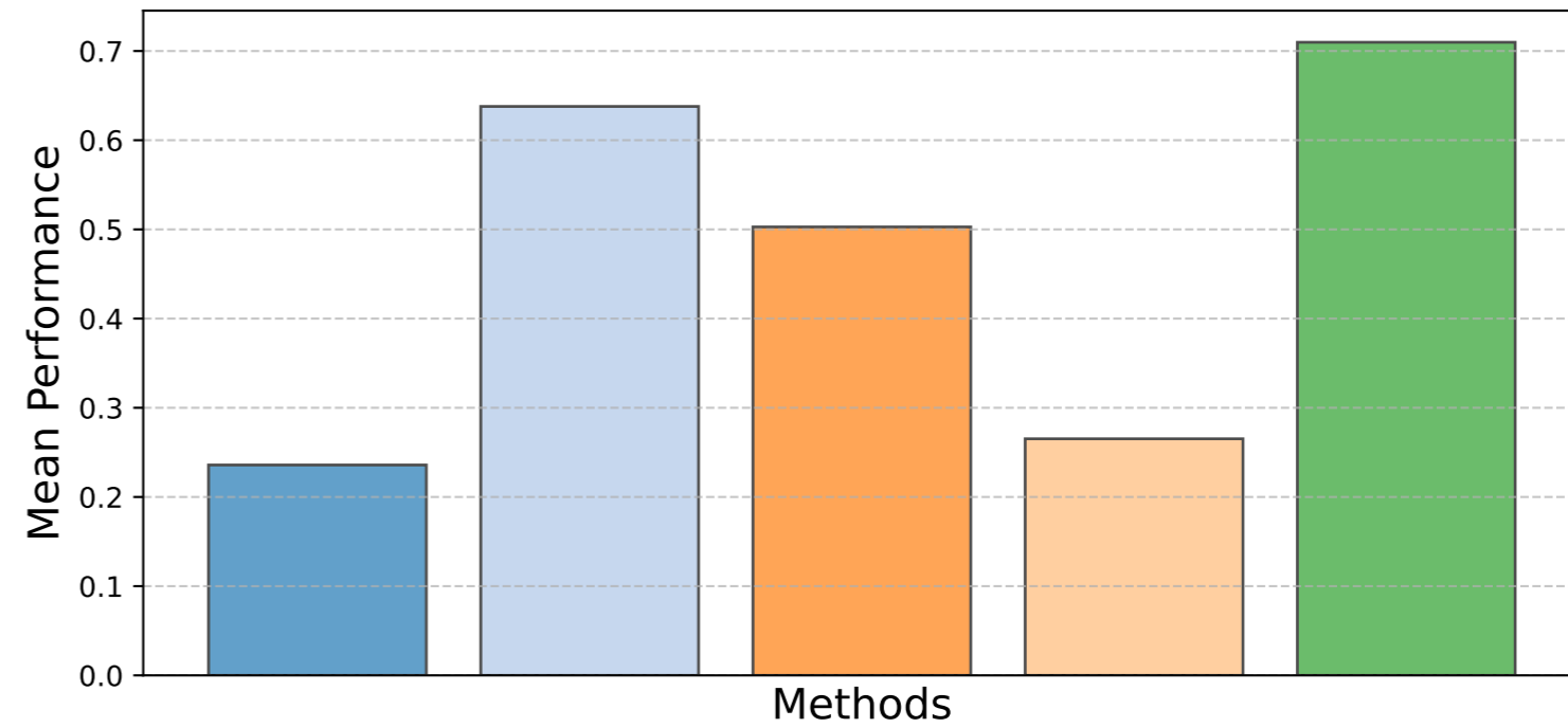
F1
