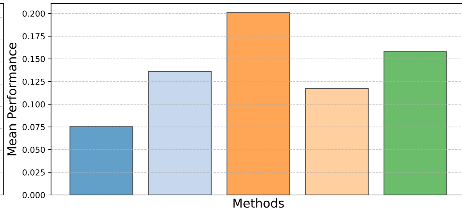
ROC AUC
