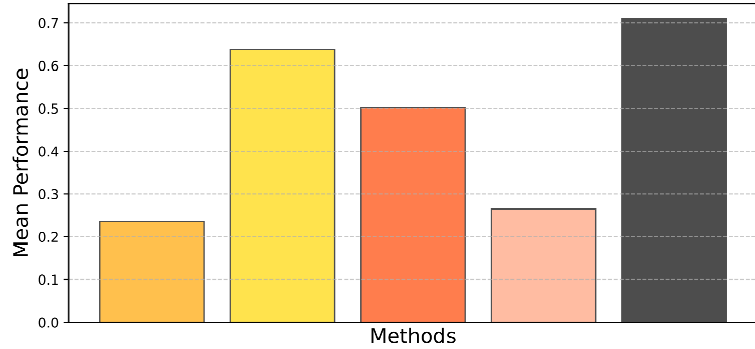
F1
