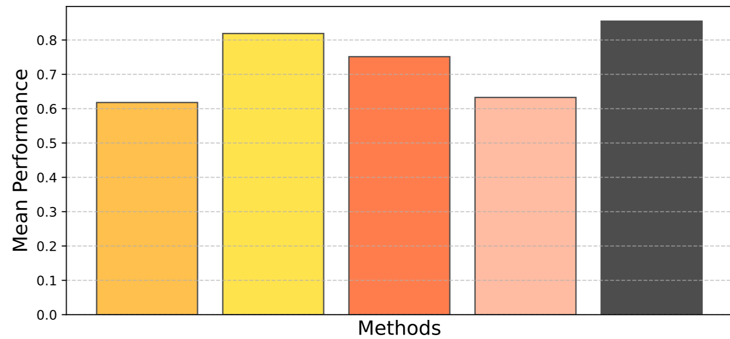
ROC AUC
