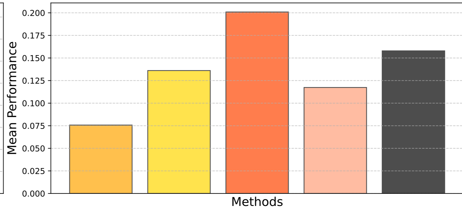
ROC AUC
